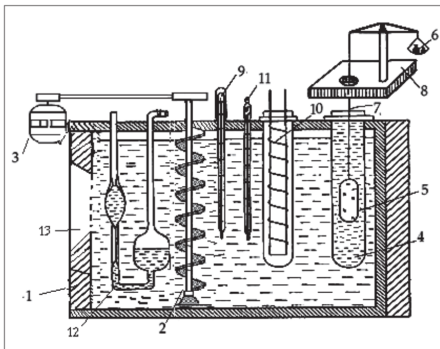
Расми 1. Сохти дастгоҳи таҷрибавӣ барои чен кардани зичӣ ва часпакии маҳлулҳо дар фишори атмосферӣ: 1 – термостат, 2 – омехтакунанда, 3 – муҳаррики электрикӣ, 4 – камера бо маводи тадқиқшаванда, 5 – шиновараки квартсӣ, 6 – сангҳои тарозу, 7 – сими манганин, 8 – тарозуи аналитикӣ, 9 – термометри симобӣ, 10 – гармкунак, 11 – ҳароратсанҷ, 12 – вискозиметри Освальд, 13 – мурипча (дастгоҳи профессор И. Ф. Голубев).
