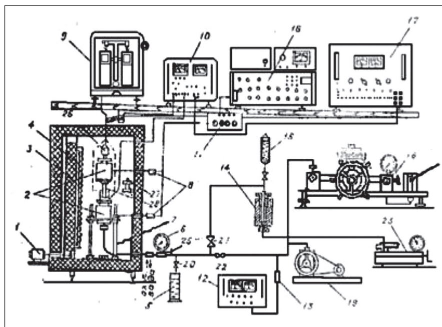
Расми 2. Дастгоҳи таҷрибавӣ барои чен кардани зичии моеъҳо ва буғҳои онҳо дар ҳаҷми сершавӣ (дастгоҳи профессор К. Д. Гусейнов ва шогирдонаш).
